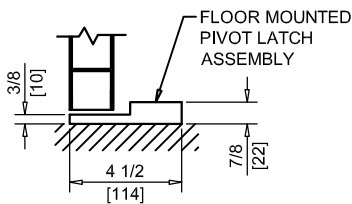
PIVOT LATCH
